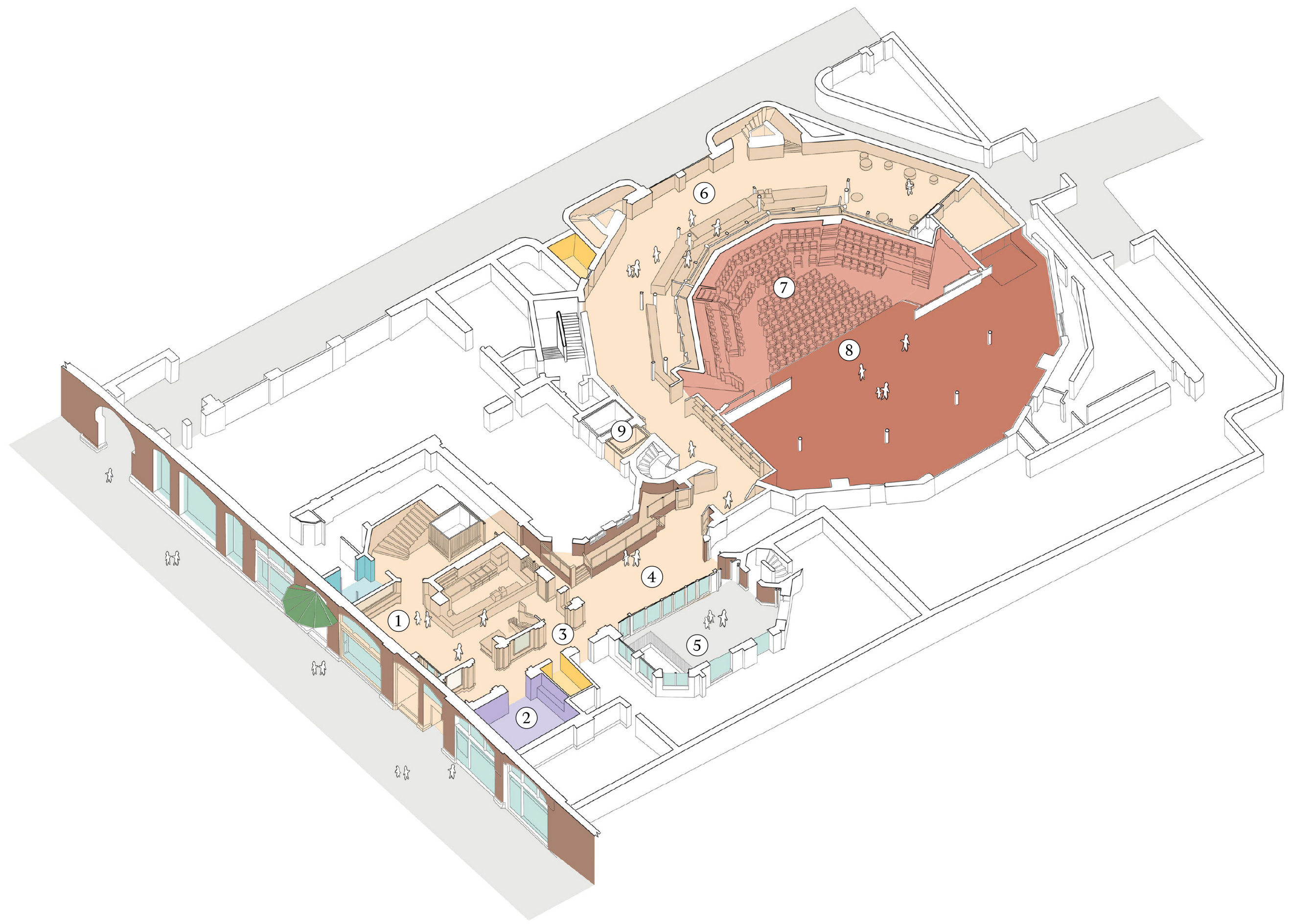
MALMÖ STADSTEATER HIPPODROMEN 2023 Level 1 Axonometric
