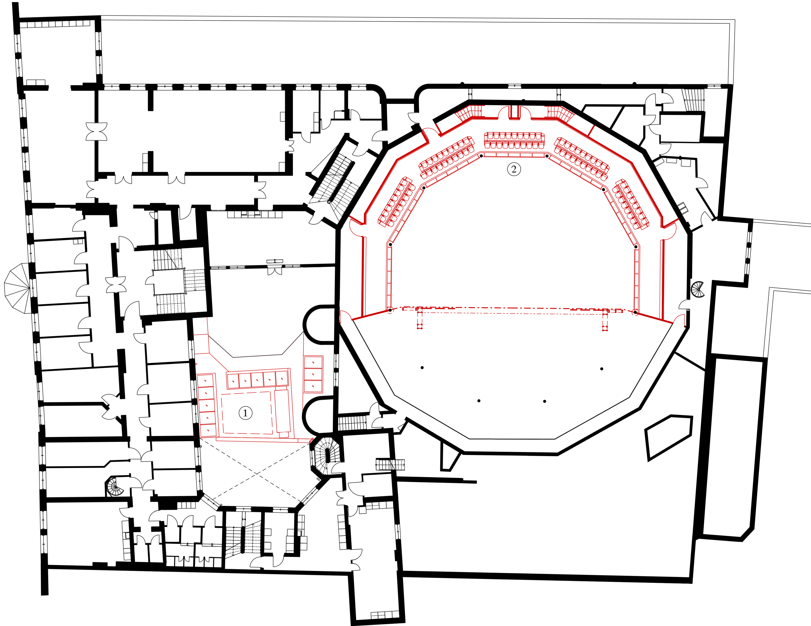
MALMÖ STADSTEATER HIPPODROMEN 2023 Level 3 Plan
